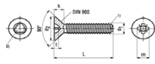
Flat Pozidriv® Type M
