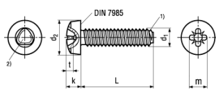
Pan Pozidriv® Type C
