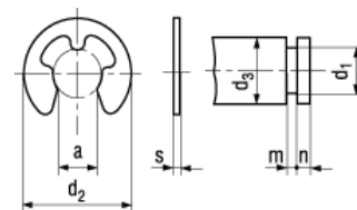
DIN 6799 Clips For Grooved Shafts
