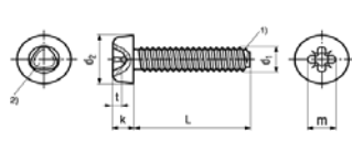
Cheese Pozidriv®
