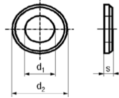
DIN 125B / ISO 7090 With Chamfer Or Radius
